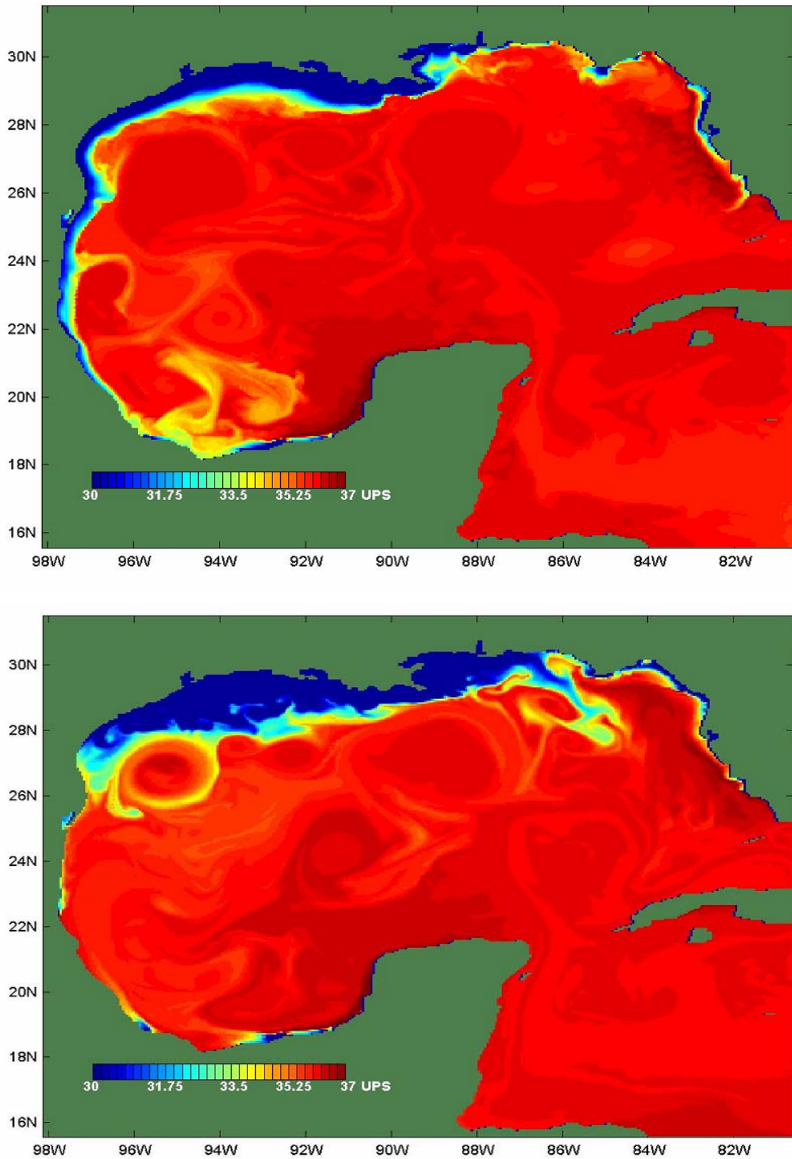
Figura 5.2 Salinidad. Mes de Enero (arriba), Julio (abajo).
