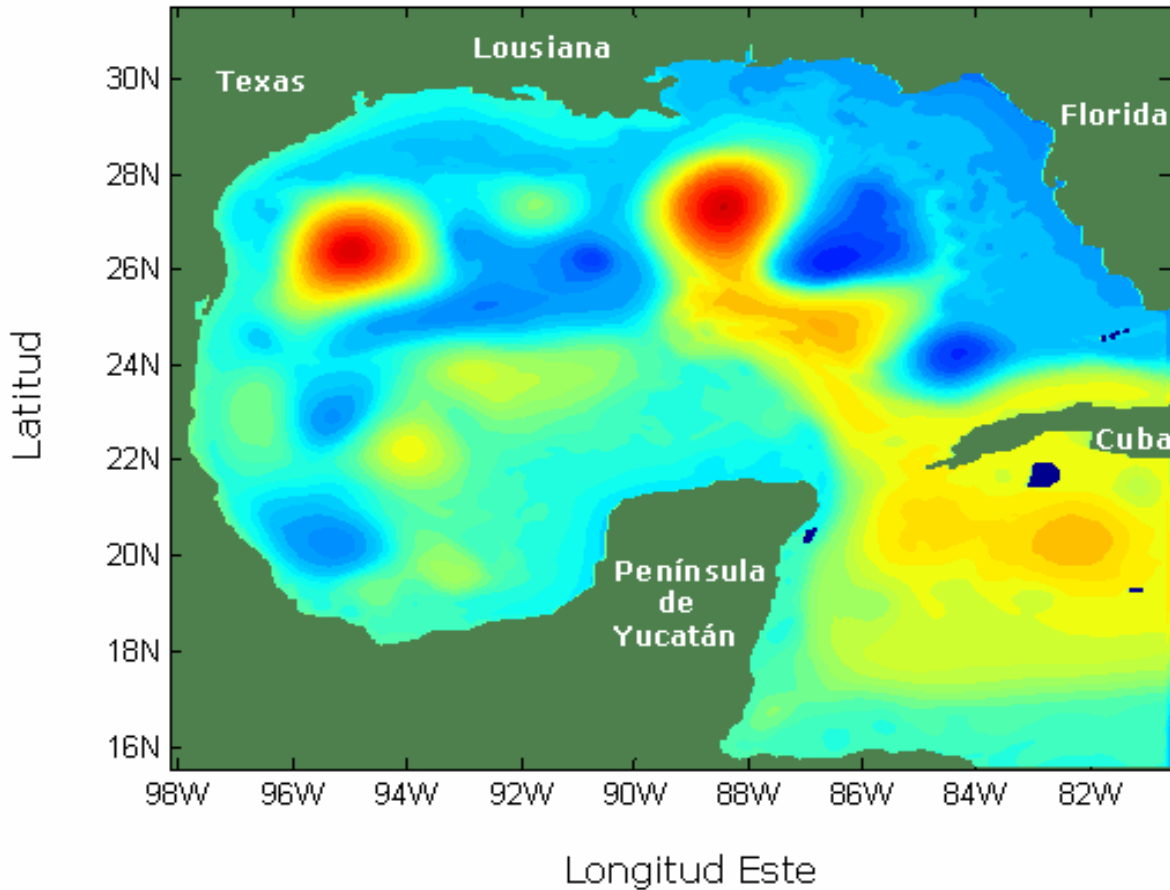
Figura 3.5 Simulación realizada con el NCOM en el Golfo de México. Se muestra el dominio del modelo.
